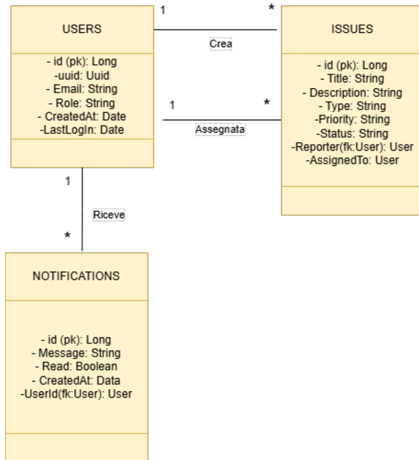
Figura 14: Schema architetturale 3 - Diagramma UML Database
