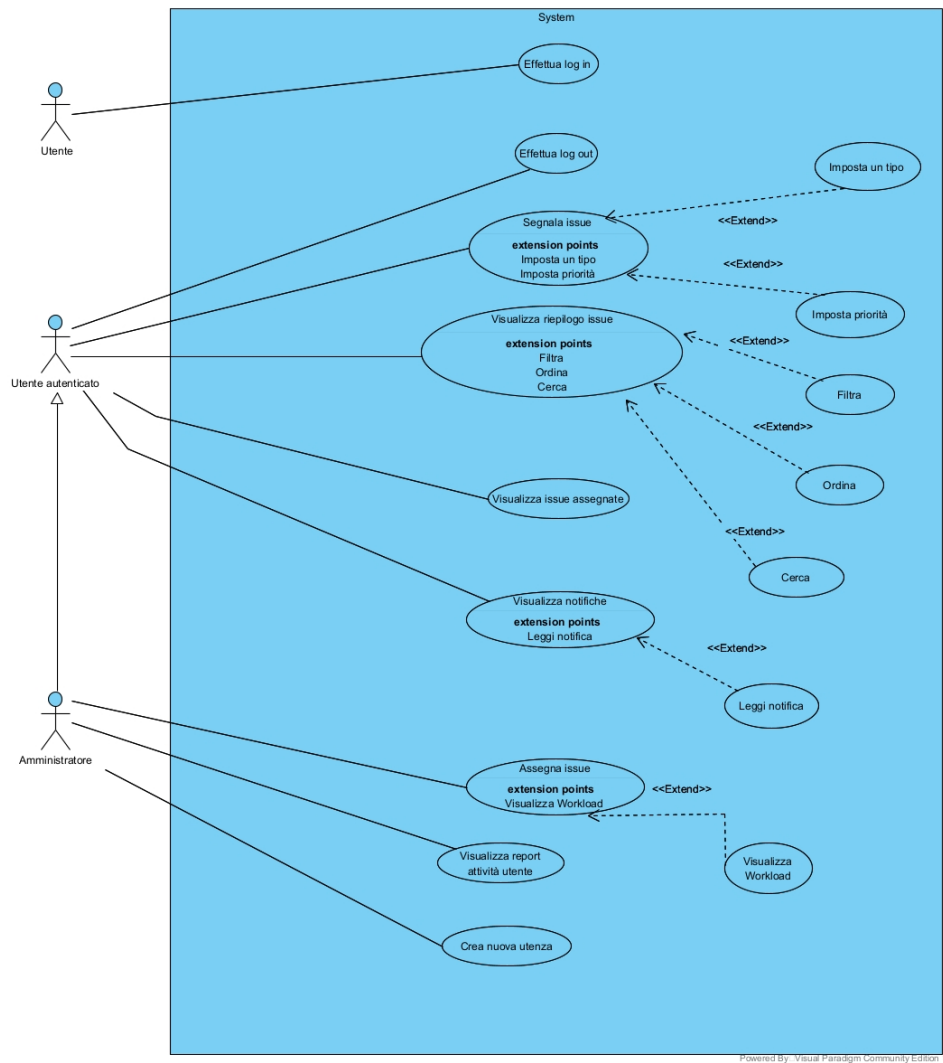
Figura 2: Use Case1 - Requisito funzionale 3.1.1 - Log in utente e Requisito funzionale 3.1.2 - Crea nuova utenza
